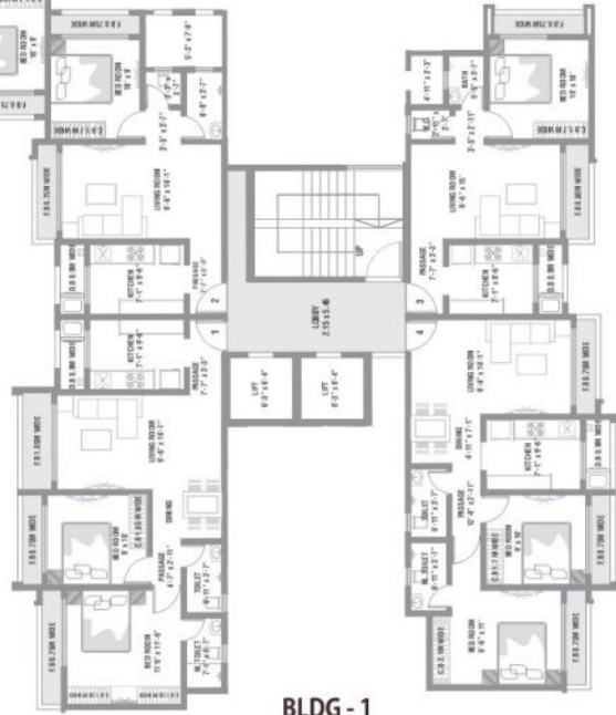
BLDG - 1
